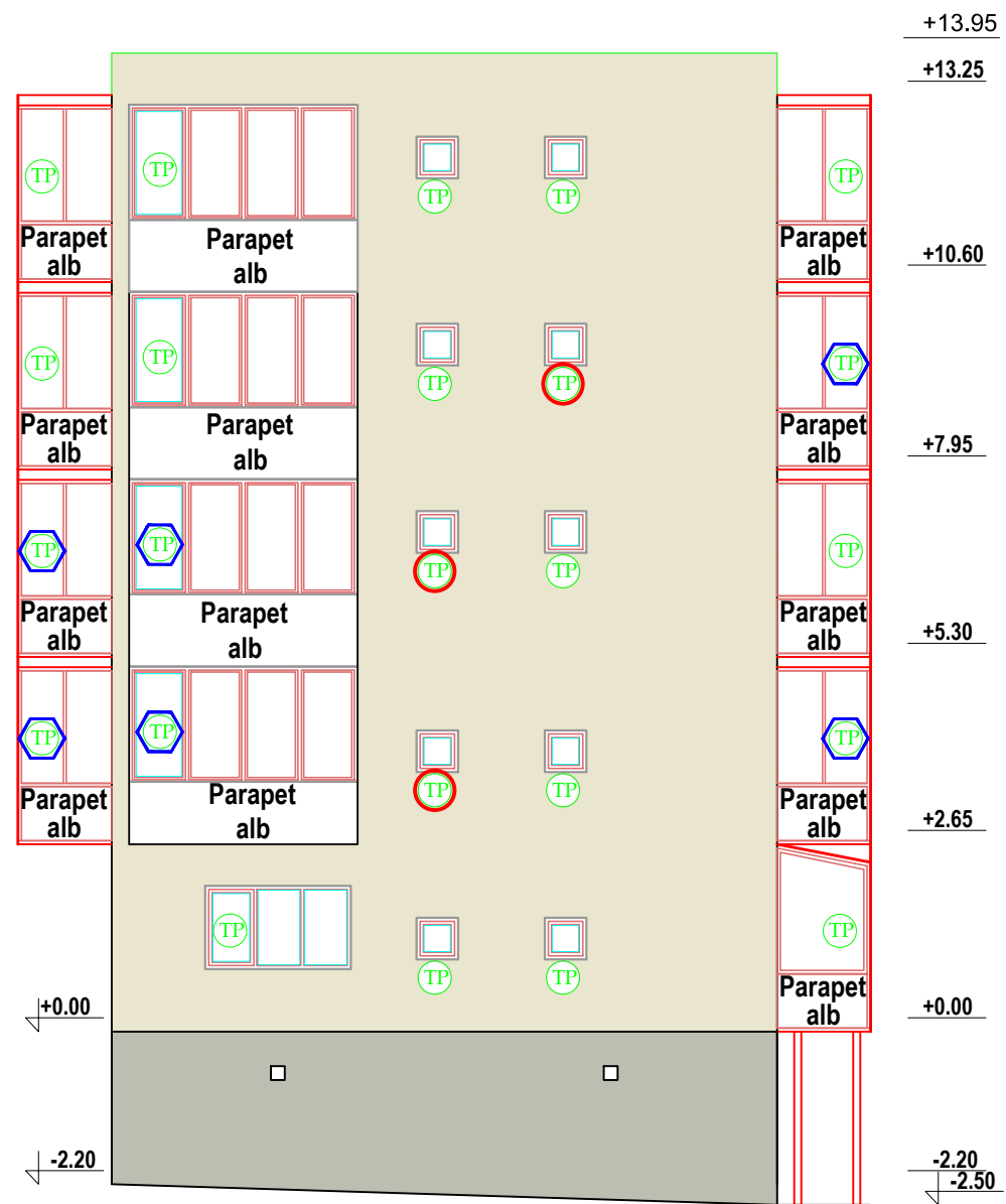
Fatada laterala dr propusa
